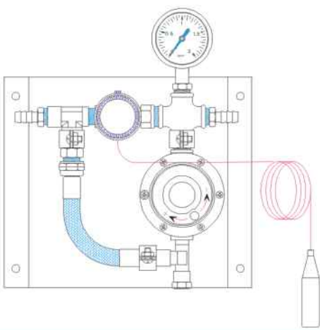
Quadro central para controle coletivo com cápsula termostática
