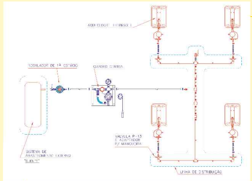
Lay-out para instalação coletiva
